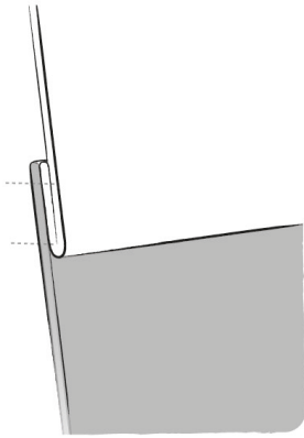
Costura plegada simple
