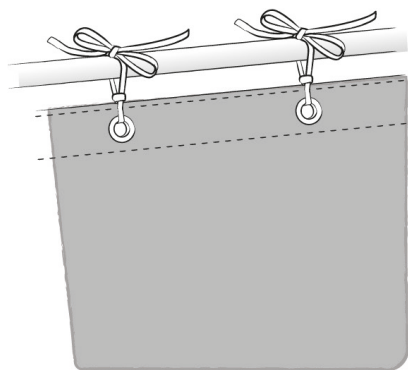
Cinta de refuerzo con ojales y cintas para atar
