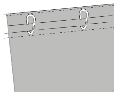
Cinta de refuerzo con mosquetones cosidos
